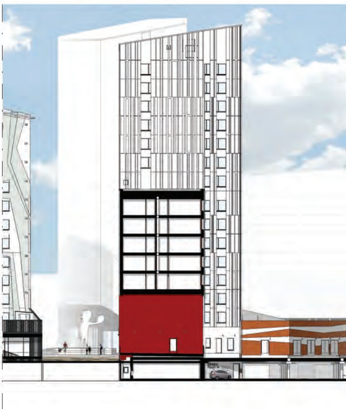
Julkisivu pohjoiseen 1:400
